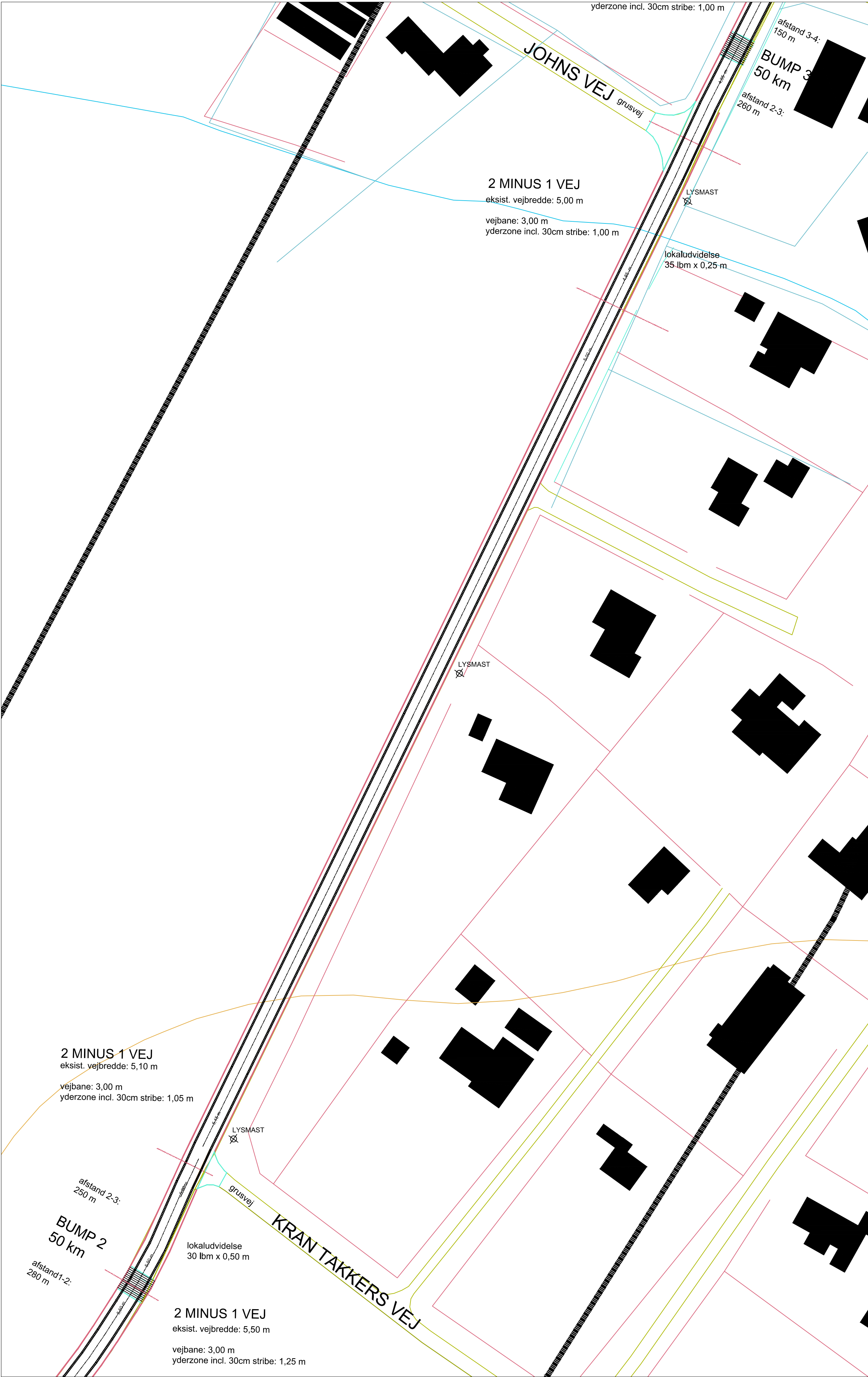
VANGSÅVEJ PLANUDSNIT 03
