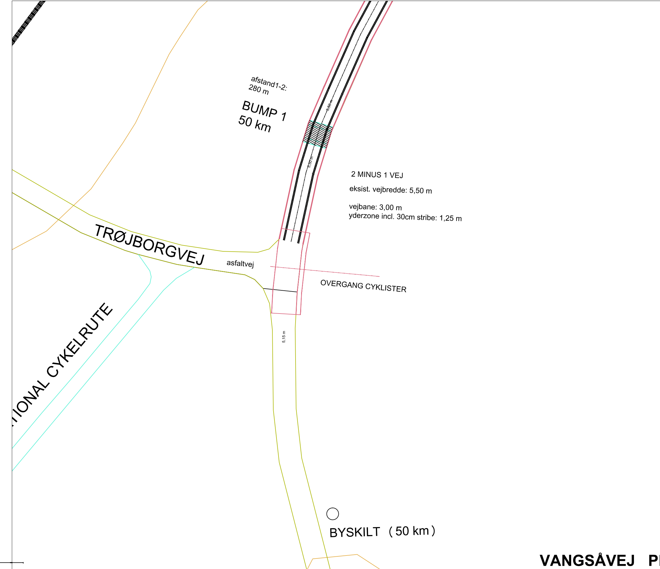
VANGSÅVEJ PLANUDSNIT 04
